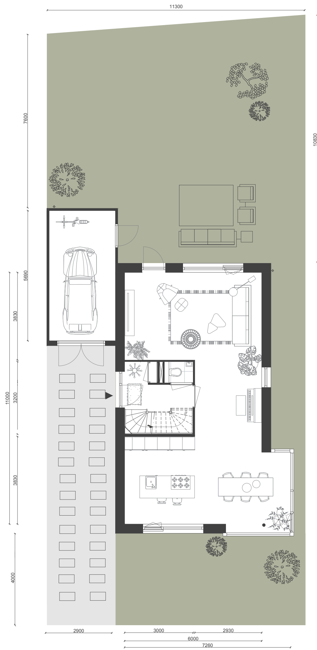
begane grond SCHAAL 1:100
