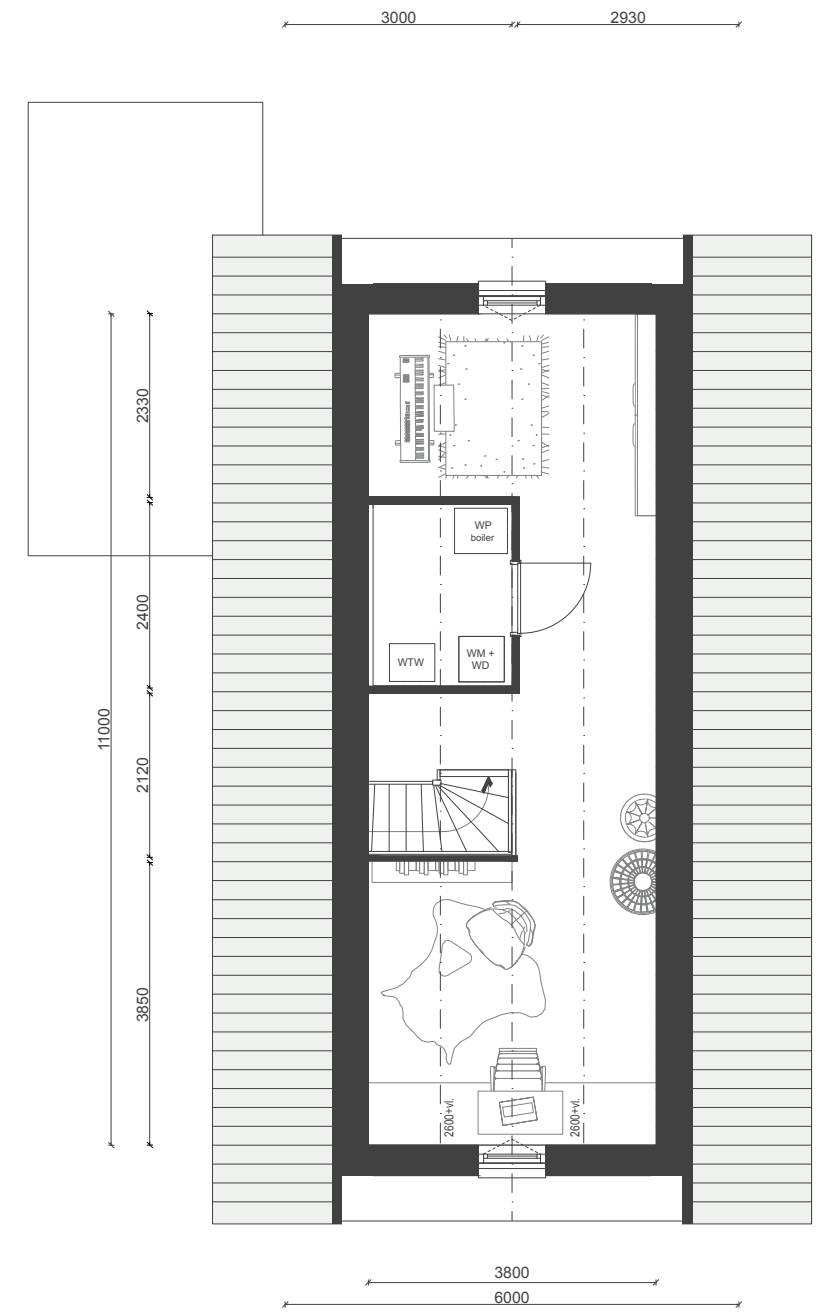
2e verdieping
